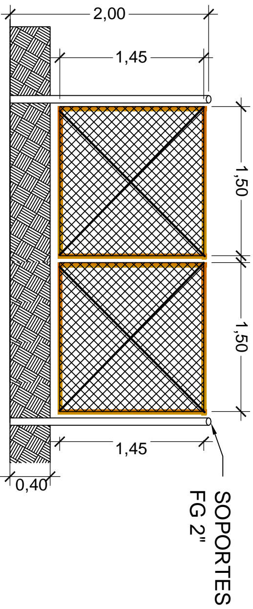
DETALLE DE LA PUERTA DE MALLA OLIMPICA
